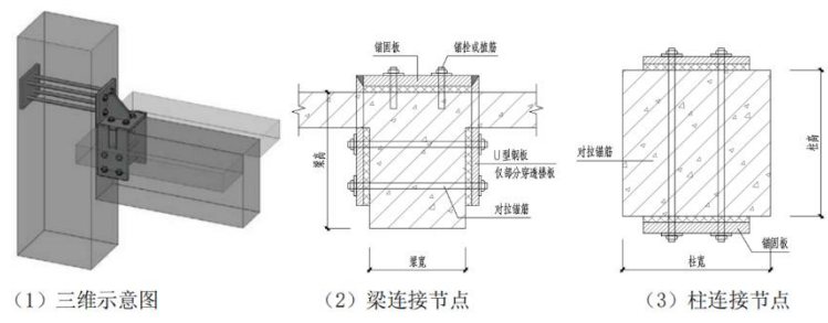
图 6.1.18-2 对拉锚固连接方法
