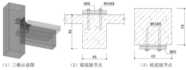
图 6.1.18-3 直接锚固连接方法
